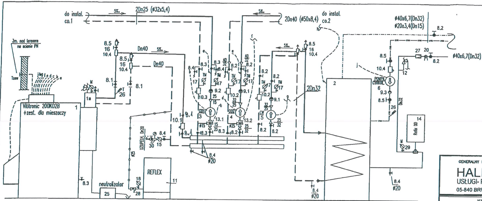
KOCIOŁ OLEJOWY VITORONDENS 200T-40 Viessmann Q=40kW
